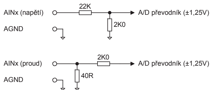
Obr. 1. Zjednodušené schéma vnitřních obvodů analogových vstupů.
