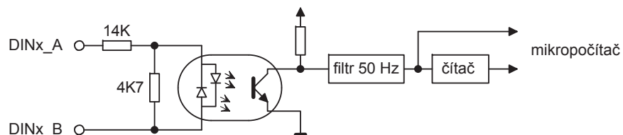
Obr. 2. Zjednodušené schéma vnitřních obvodů digitálních vstupů.
