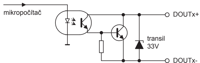
Obr. 3. Zjednodušené schéma vnitřních obvodů digitálních výstupů.
