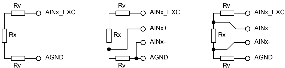
Obr.3. Zjednodušené schéma připojení odporových čidel (dvou, tři a čtyřvodičová topologie; rezistory Rv znázorňují odpor přívodních vodičů).
