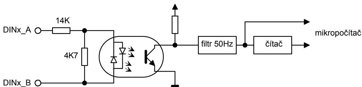
Obr.4. Zjednodušené schéma obvodů digitálních vstupů.
