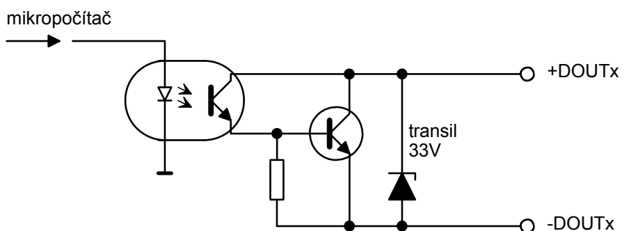
Obr.5. Zjednodušené schéma obvodů digitálních výstupů MU-415/815.
