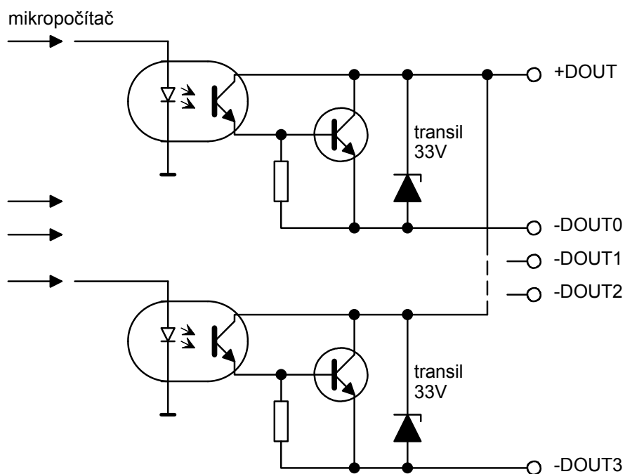
Obr.6. Zjednodušené schéma obvodů digitálních výstupů MU-416/816.
