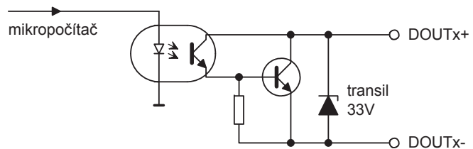
Obr. 1. Zjednodušené schéma vnitřních obvodů digitálních výstupů.
