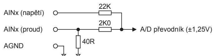
Obr. 1. Zjednodušené schéma vnitřních obvodů analogových vstupů.
