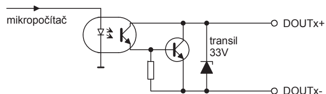
Obr. 3. Zjednodušené schéma vnitřních obvodů digitálních výstupů.
