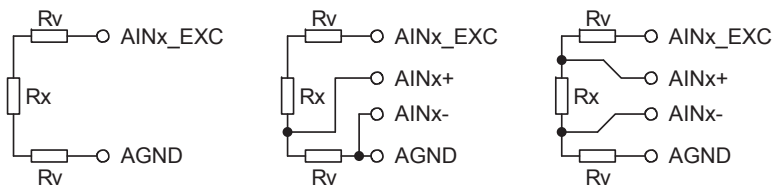
Obr. 1. Schéma připojení odporových čidel (dvou, tři a čtyřvodičová topologie; rezistory R_v znázorňují odpor přívodních vodičů).
