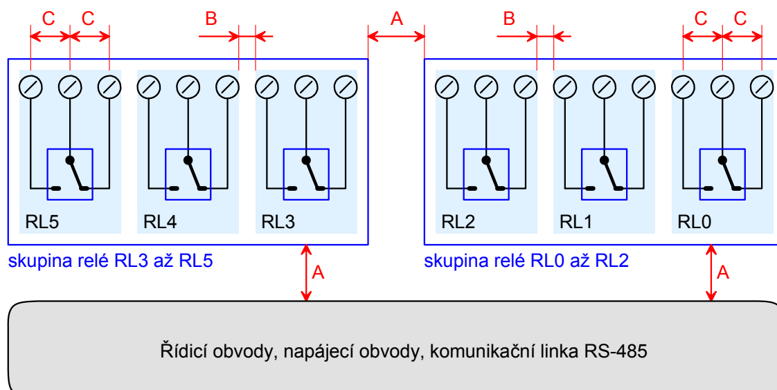
Obr.2. Zjednodušené schéma vnitřních obvodů reléových výstupů.
