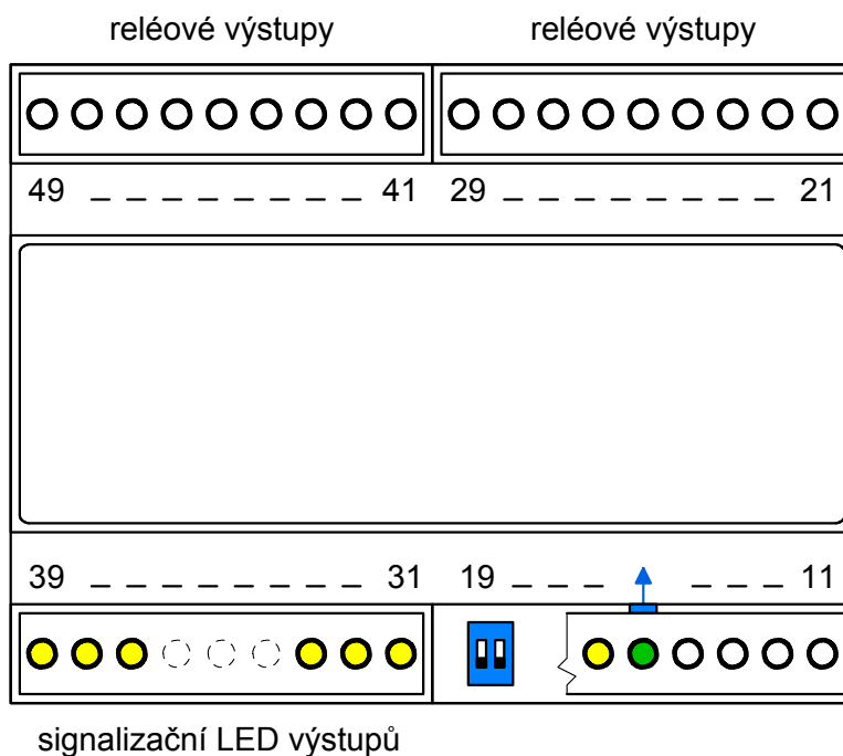
Obr.1. Obrázek modulu MU-653.
