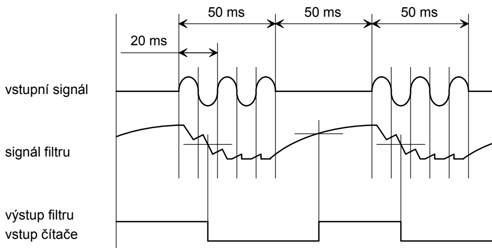
Obr.3. Dolnoproputný filtr 50 Hz. V případě modulu MU-826 je potřeba, aby signál 50 Hz byl aktivní po dobu alespoň 50 ms a neaktivní po dobu rovněž alespoň 50 ms. Maximální frekvence na výstupu filtru tedy může dosáhnout 10 Hz.
