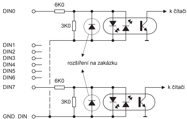
Obr. 1. Zjednodušené schéma vstupních obvodů modulů.
